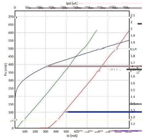
785nm P-I-V
