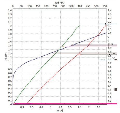
808nm P-I-V
